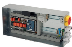
rozvaděč Digireg® evo.018
