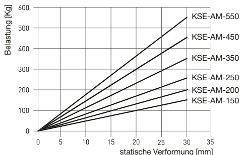
statische Verformung
