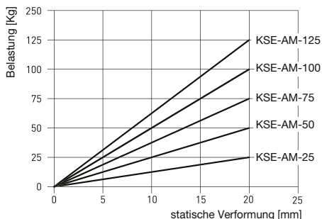
statische Verformung
