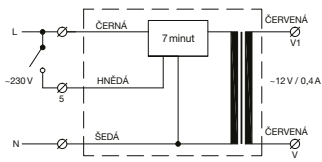
vnitřní zapojení CTE 12/708
