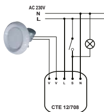
zapojení CTE 12/708 s KEL
