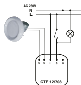
Verbindung CTE 12/708 mit KEL
