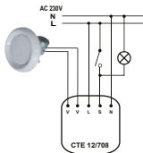
Verbindung CTE 12/708 mit KEL
