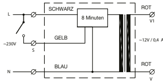
interne Verkabelung CTE 12/708
