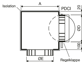
Anschlusskasten PDC / PDCI
