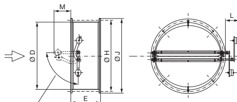
TSK BR 630–1250 (pouze vodorovně)
