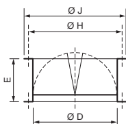
TSK BR 400–560 (svisle i vodorovně)
