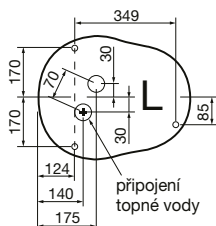
připojení topné vody
