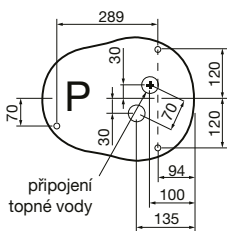
DOR-V-W rozměry připojení s vodním ohřevčem
