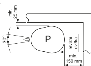
minimální odstupy od konstrukcí
