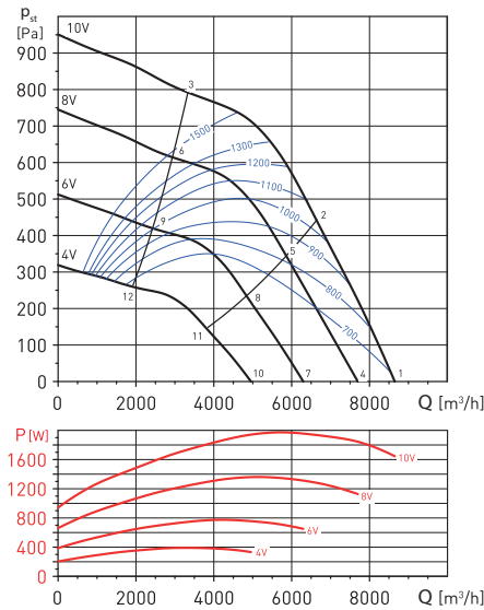
KABT-9000/500 Ecowatt
