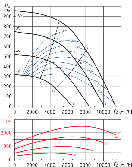
KABT-12000/560 Ecowatt
