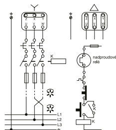
zapojení Y nebo Δ podle typu a štítku na motoru
