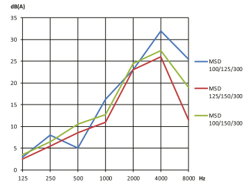
Einfügungsdämpfung
