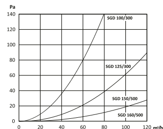
tlaková strata
