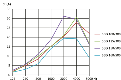
vložný útlum
