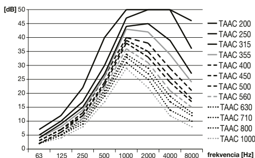
Útlm tlmičov TAAC
