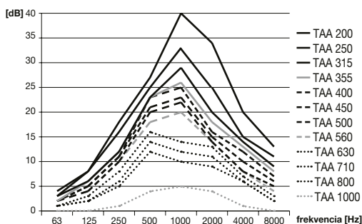
Útlm tlmičov TAA
