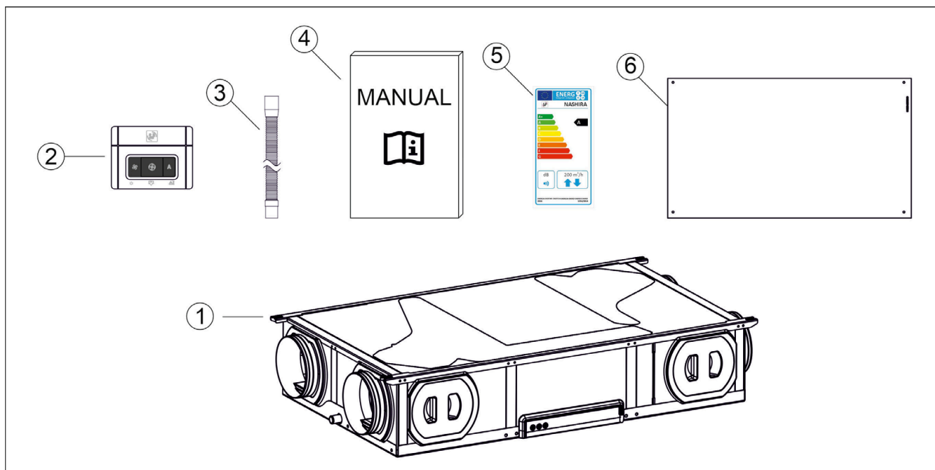
Obrázek 1. Dodávané součásti
