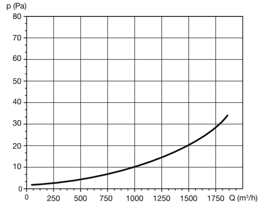
Druckverlustwerte des Dachkopfes VH 315 abhängig von der Luftströmung im Druckrohr (Richtwerte)
