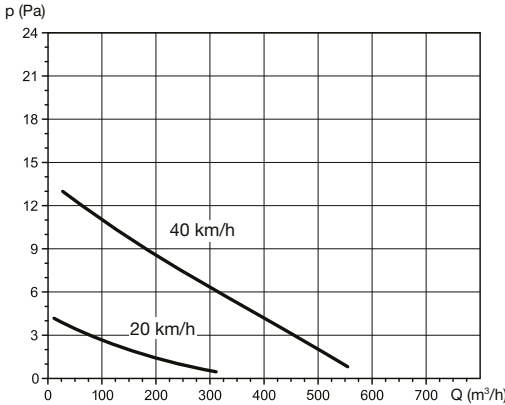
Druckverhalten des Dachkopfes VH 315 abhängig von der Windgeschwindigkeit (Richtwerte)
